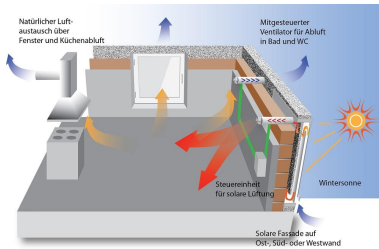
Die Funktionsweise des solaren Lüftungssystems SunAir
